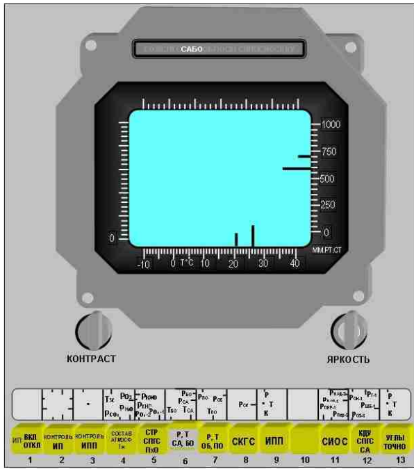
Рис. 2.1.5 Формат отображения «Давление, температура в СА, БО»
