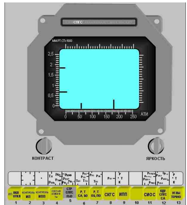
Р о2 -1, Р о2 -2, датчик «ДТ-250 С, диапазон измерения 0 – 250 АТИ Р юко , Р кнр , датчик МДДАС-100-2300, диапазон измерения 100 – 2300 мм.рт.ст.
