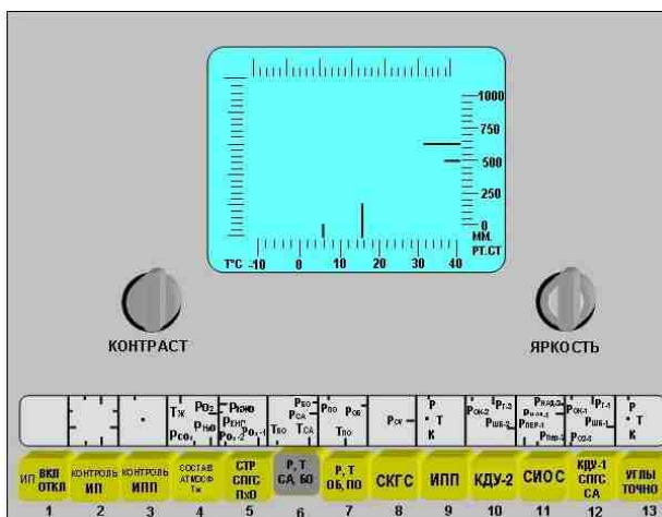
Рис.2.2.5 Вид формата отображения «Давление и температура в СА и БО»
