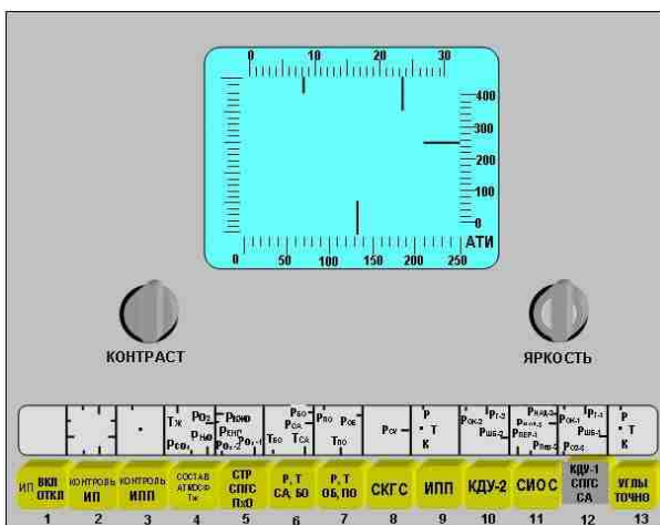
Рис.2.2.11 Вид формата отображения «КДУ, СПГС, СА»
