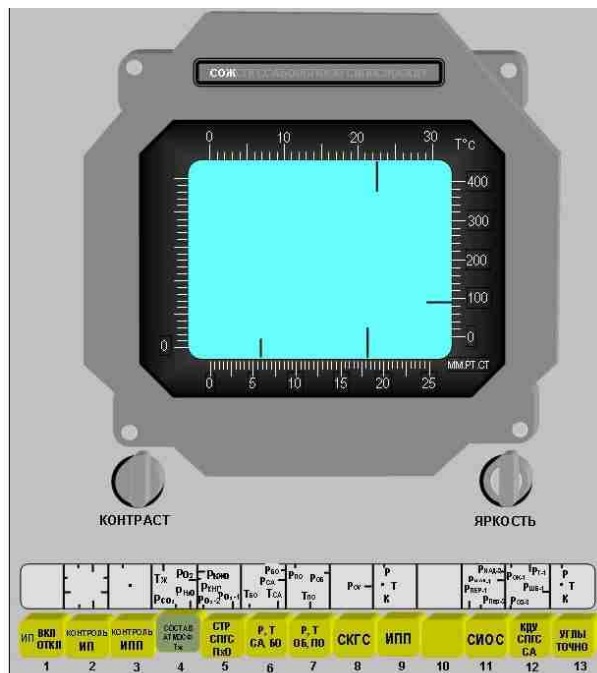
Параметры: Р о2 - 0 – 350 мм.рт.ст, датчик КМ 0 305М, сигнал 0 – 6,2 В Р со2 - 0 – 25 мм.рт.ст, датчик КМ 0 305М, сигнал 0 – 6,2 В Р Н2О - 5– 15 мм.рт.ст, датчик КМ 0 305М, сигнал 0 – 6,2 В Т ж - 0 - 20°С, датчик ДТЖ 1А, терморезистор
