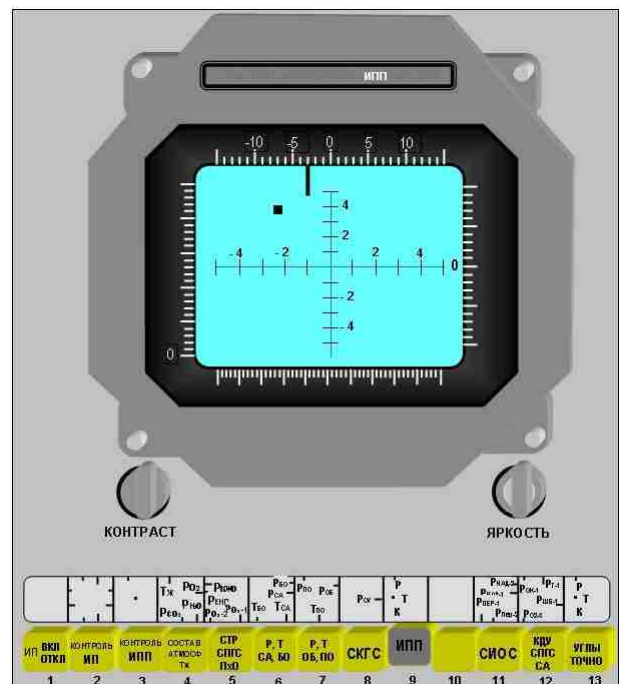
Рис. 2.1.8 Вид формата отображения «Индикация параметров положения осей корабля относительно базовой орбитальной системы координат».
