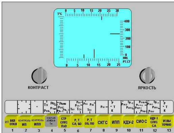
Рис.2.2.3 Вид формата отображения «Состав атмосферы»
