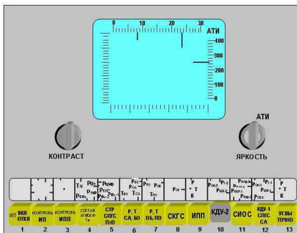
Рис. 2.2.9 Вид формата отображения «КДУ2»
