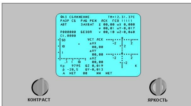
Рис. 2.2.13 Вид формата отображения 43 «СБЛИЖЕНИЕ», формируемый БФИ аппаратуры «Символ».
