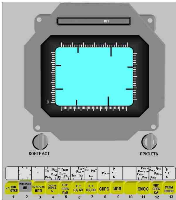
Рис.2.1.1 Вид формата отображения «Контроль измерения параметров». Контроль работы КЗИ (ВКУ, ШУ, формирова- тель изображения аппаратуры «Стрелка-ВМ», блок телевизионной системы (коммутатор)
