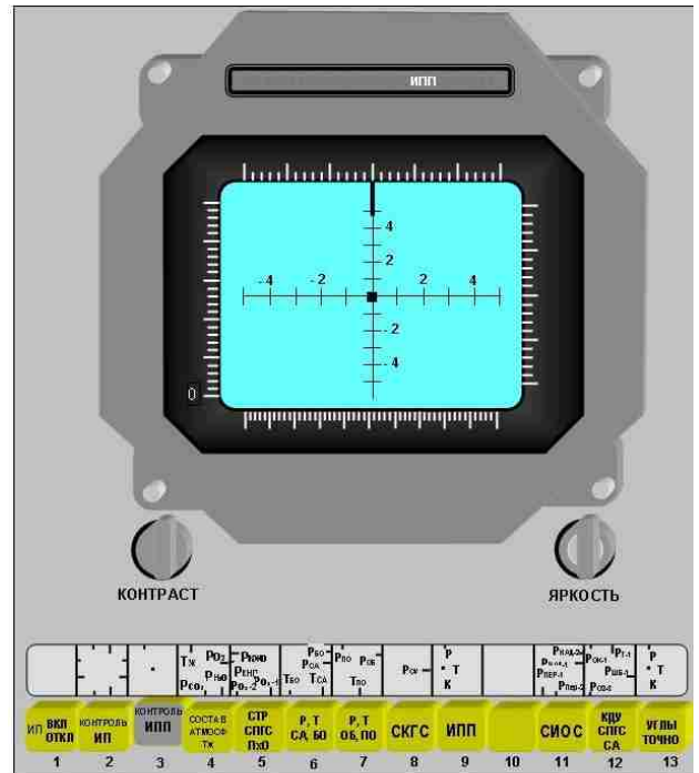
Рис. 2.1.2 Вид формата отображения «Контроль измерения параметров положения осей корабля относительно базовой орбитальной системы координат».
