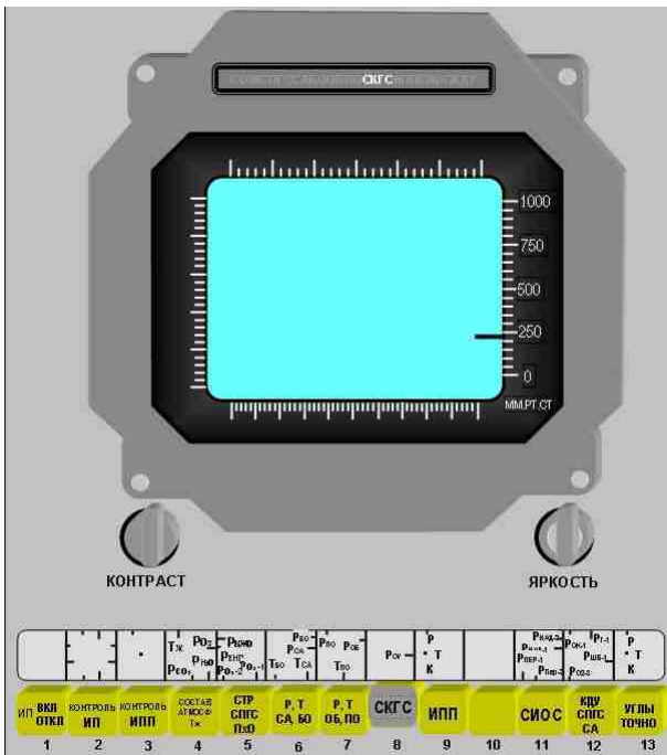
Рис. 2.1.7 Формат отображения системы контроля герметичности стыка «Давление»
