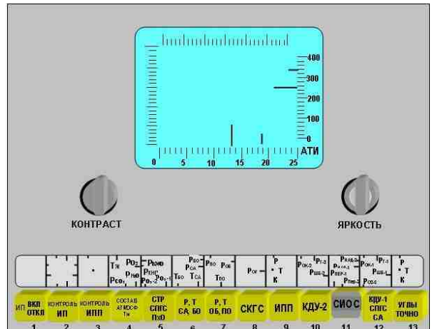
Рис.2.2.10 Вид формата отображения «СИОС»
