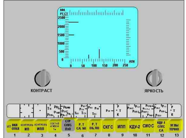
Рис. 2.2.4 Вид формата отображения «давление в СТР, СПГС, ПхО»
