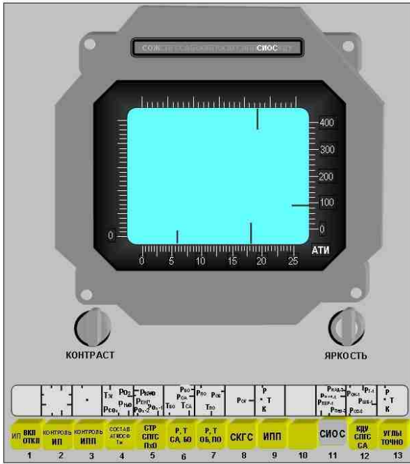
Рис.2.1.9 Вид формата отображения «СИОС»
