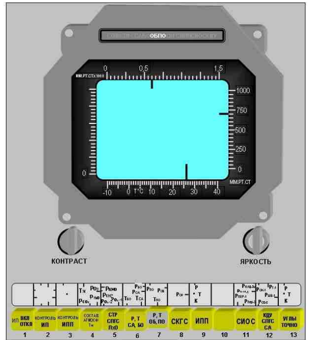
Рис. 2.1.6 Формат отображения «Давление, температура в ОБ, ПО»
