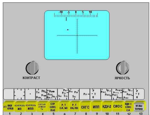
Рис.2.2.12 Вид формата отображения «УГЛЫ ТОЧНО»
