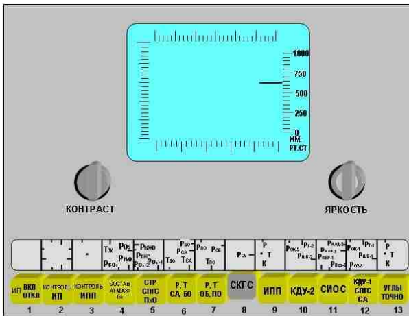
Рис. 2.2.7 Вид формата отображения «СКГС»
