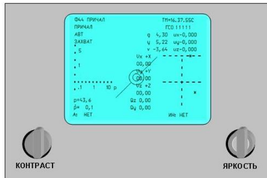
Рис. 2.2.14 Примерный вид формата отображения «ПРИЧАЛИВАНИЕ», формируемый БФИ аппаратуры «Символ».
