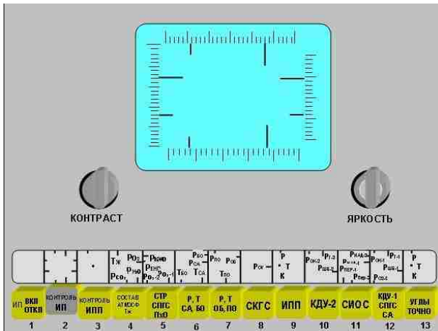
Рис.2.2.1 Вид формата отображения «Контроль измерения параметров». Контроль работы КЭИ (ВКУ, ШУ, формирователь изображения аппаратуры «Стрелка-ВМ», блок телевизионной системы (коммутатор))
