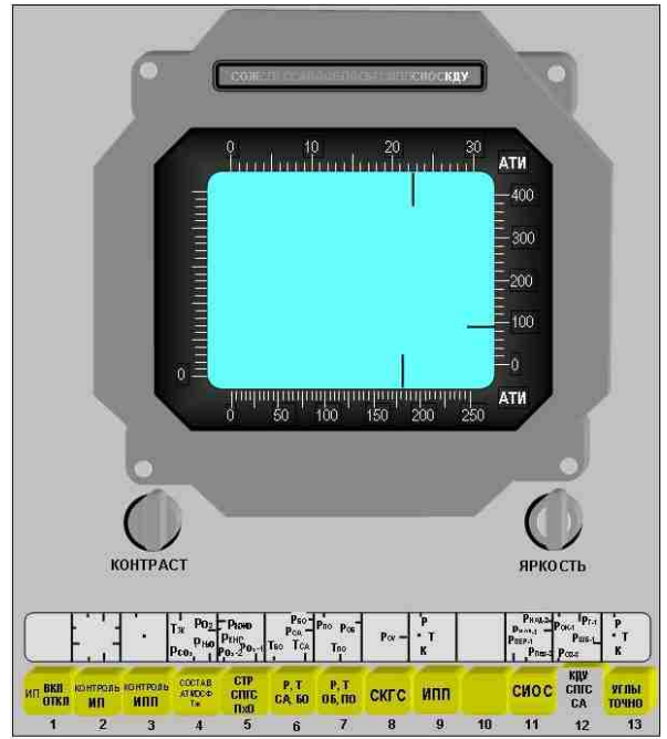
Рис. 2.1.10 Вид формата отображения «КДУ, СПГС, СА»
